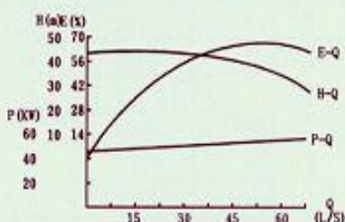
ZW150-180-38
