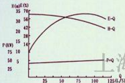
ZW200-280-28
