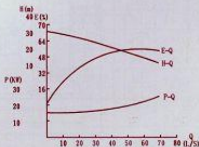
ZW150-180-20
