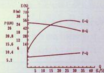
ZW150-180-20
