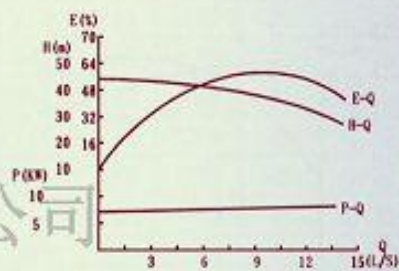
ZW65-25-40
