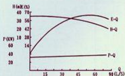
ZW150-180-30
