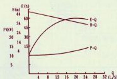
ZW80-80-35
