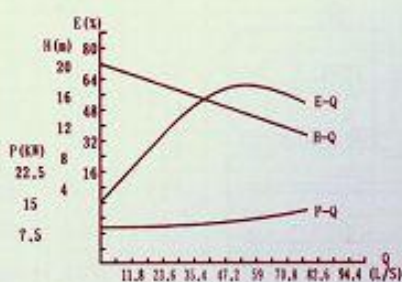
ZW150-180-14
