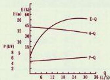
ZW100-100-15
