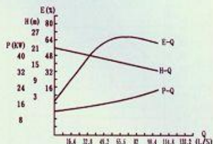
ZW200-280-14
