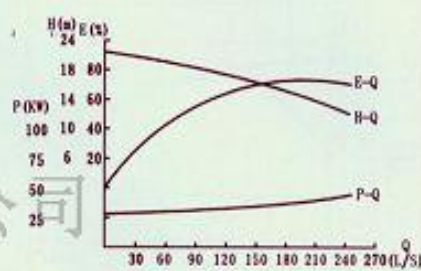
ZW300-800-14
