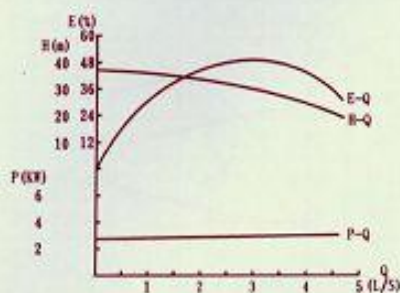
ZW32-9-30
