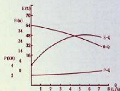
ZW40-15-30 ZW50-15-30
